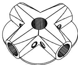
Соединитель 5 труб угловой, с 3 полками, хром.
